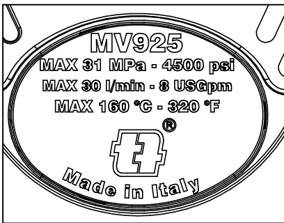
DETTAGLIO-DETAIL B
