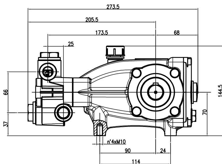
Dimensioni d' ingombro
